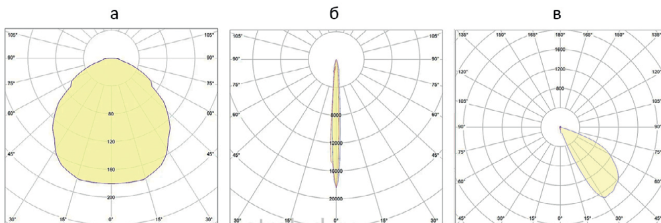
Рис. 11. Примеры КСС (а – широкий угол; б – узкий угол; в – асимметричное распределение света)
