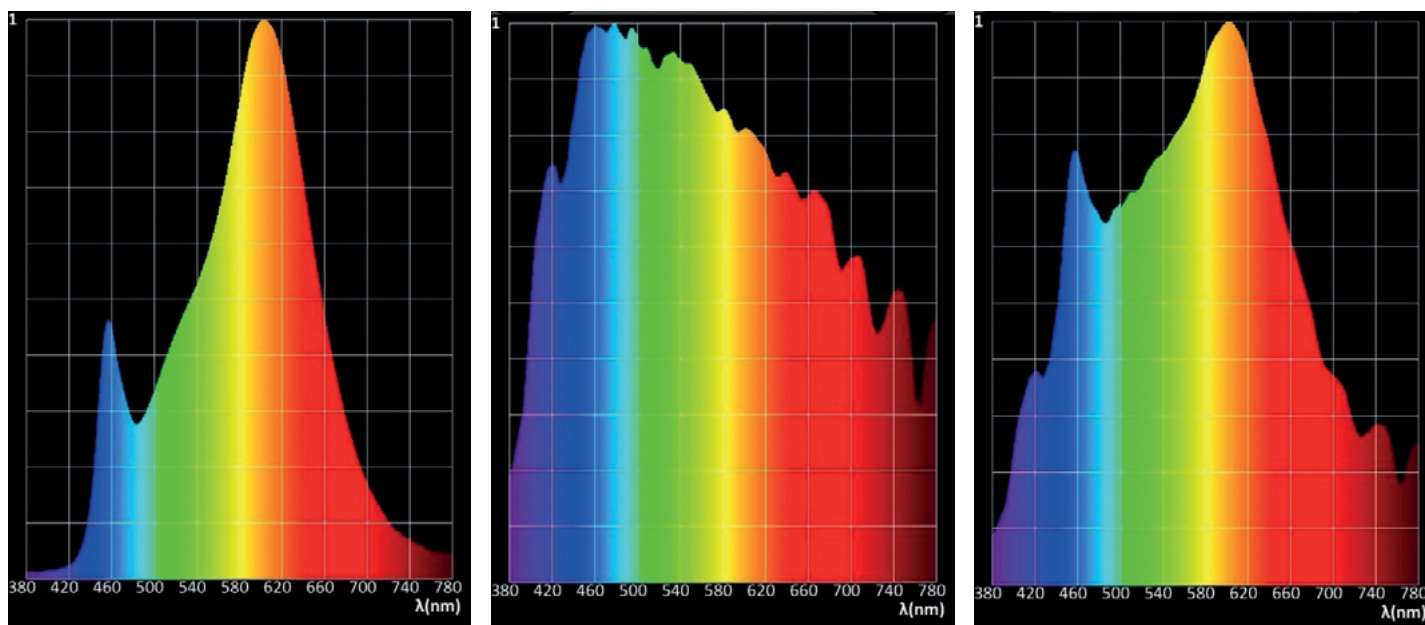
Рис. 44. Результаты измерений спектра источников света с помощью спектрометра (слева направо): правильно измеренный светодиодный источник света; солнечный спектр; искаженный (совмещенный) спектр искусственного и естественного света из-за неверного расположения прибора. На искаженном результате отчетливо видны «пики» спектра светодиода с цветовой температурой 3000 К
