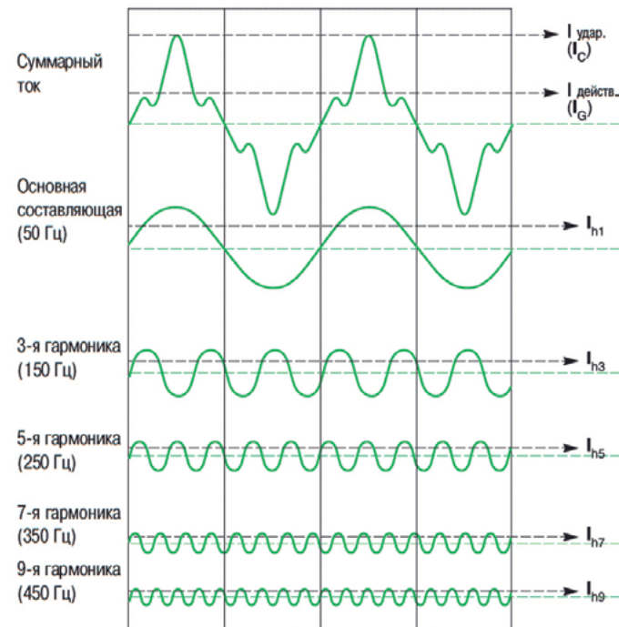
Рис. 10. Высшие гармоники первых порядков и искажение синусоиды тока фундаментальной частоты 50 Гц 7
