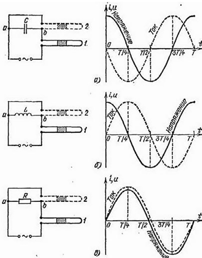
Рис. 9. Фазовые сдвиги
