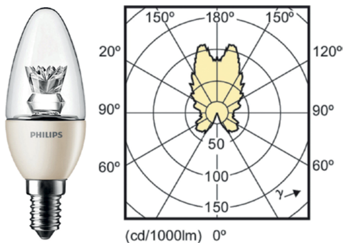
Рис. 39. Внешний вид и КСС линзованной светодиодной лампы
