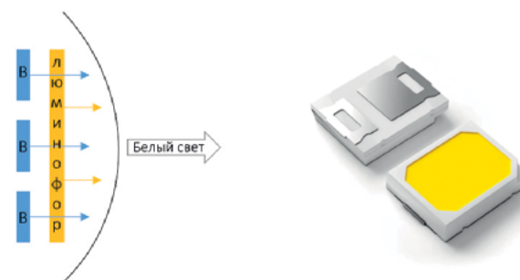
Рис. 6. Принцип действия и пример внешнего вида люминофорного СД 5
