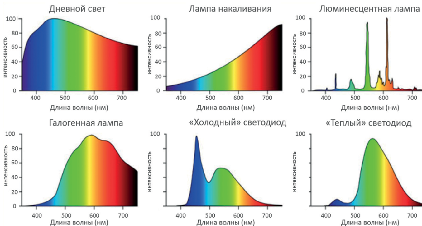
Рис. 13. Спектры излучения различных источников света в видимом диапазоне
