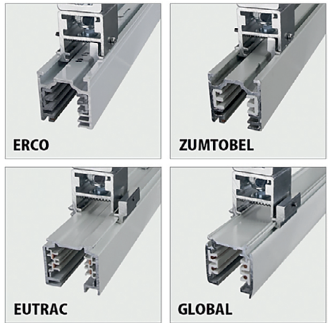
Рис.27. Трехфазные осветительные треки распространенных производителей в разрезе
