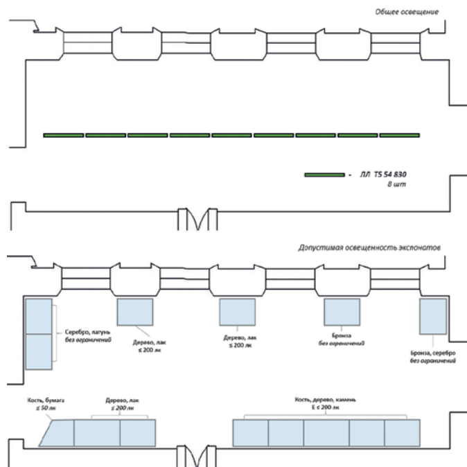
Рис. 42. Пример содержания осветительной карты зала
